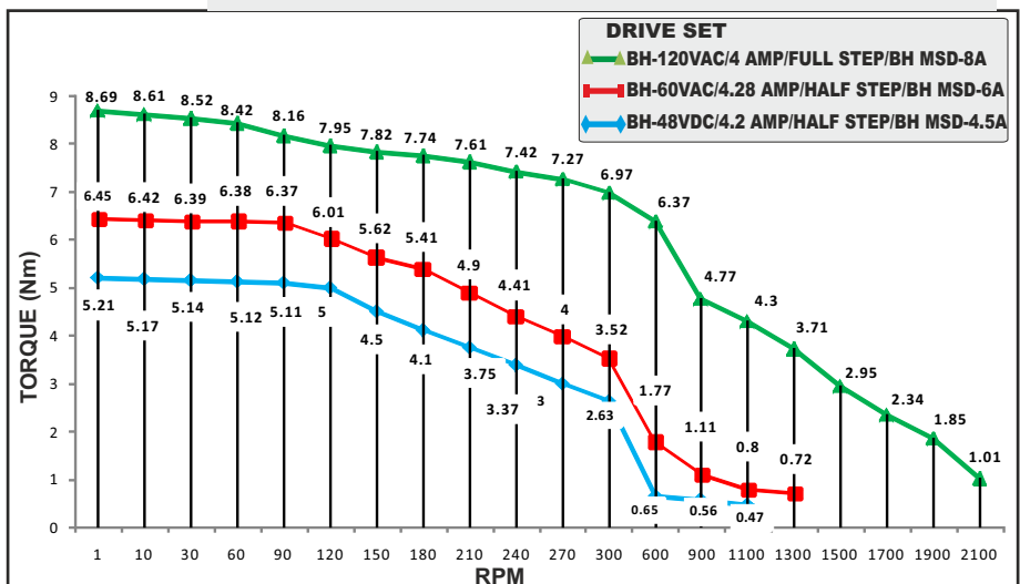
STEPPER MOTOR - BH86SH118- 4004 AKS-CE
